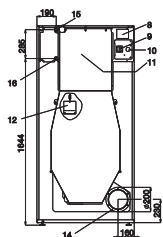
TRAZ: T 24 35 AQUECIMENTO A VAPOR
