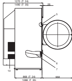
TRAZ: T 24 35 AQUECIMENTO A GÁS
